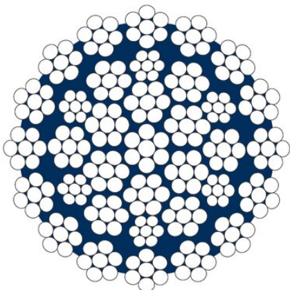
Torņa celtņiem
