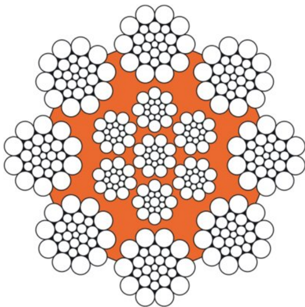
Tilta celtņiem
